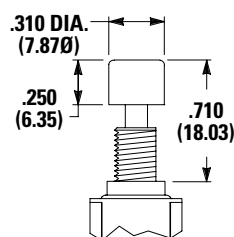
S, S1, S2, Plunger Dimensions
