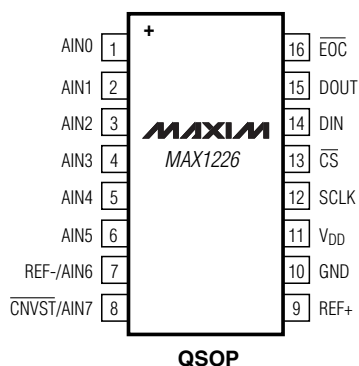
QSOP
